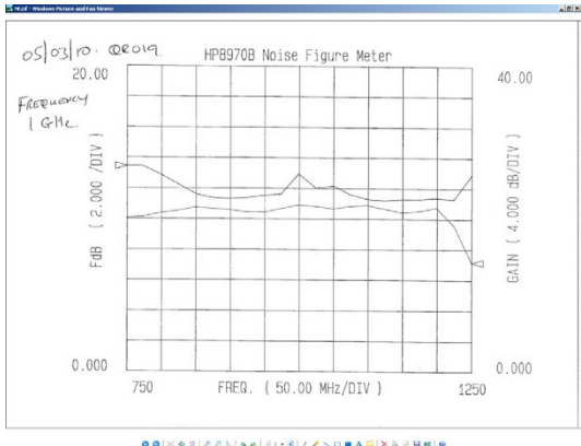
Low RF, 500MHz IF Bandwidth
