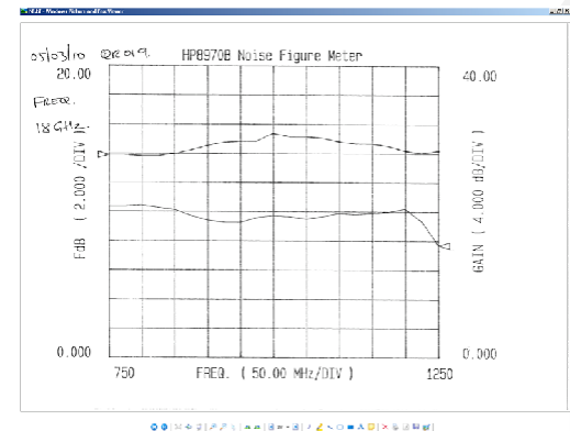
High RF, 500MHz IF Bandwidth
